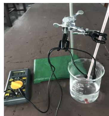
實驗裝置
