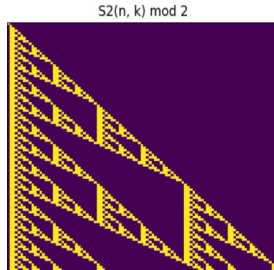
圖二： S(n, k) 的奇偶性分佈圖（本圖由作者親自製作）
