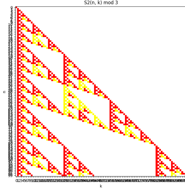
圖八：斯特靈數三角形 mod 3 （本圖由作者親自製作）
