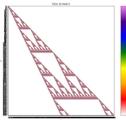
圖十三：第一類斯特靈數模 2
