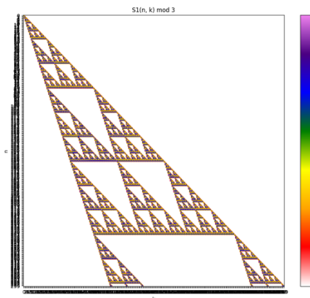
圖十四：第一類斯特靈數模 3
