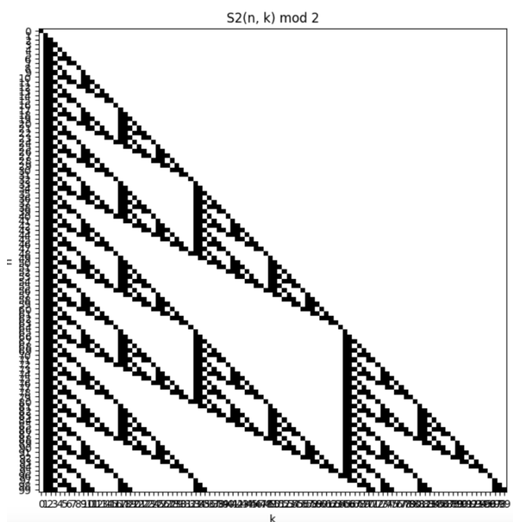
圖四： S(n, k) 的奇偶性分佈圖（黑白版，本圖由作者親自製作）
