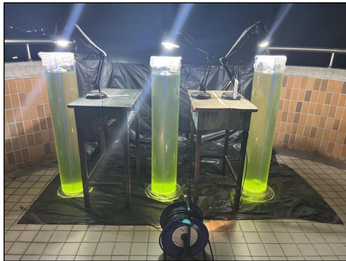
（圖 10）夜間增加照度 1800 lux 的燈源於量筒上方
