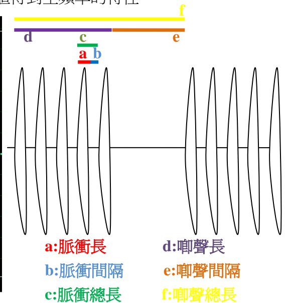
圖(八)呼喚聲波形示意圖
